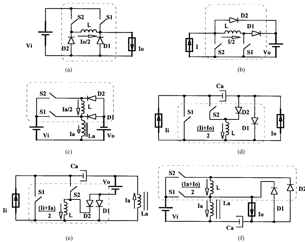
Fig. 15. The 2I dc-dc converters family: (a) buck, (b) boost, (c) buck-boost, (d) cuk, (e) sepic, and (f) zeta.
